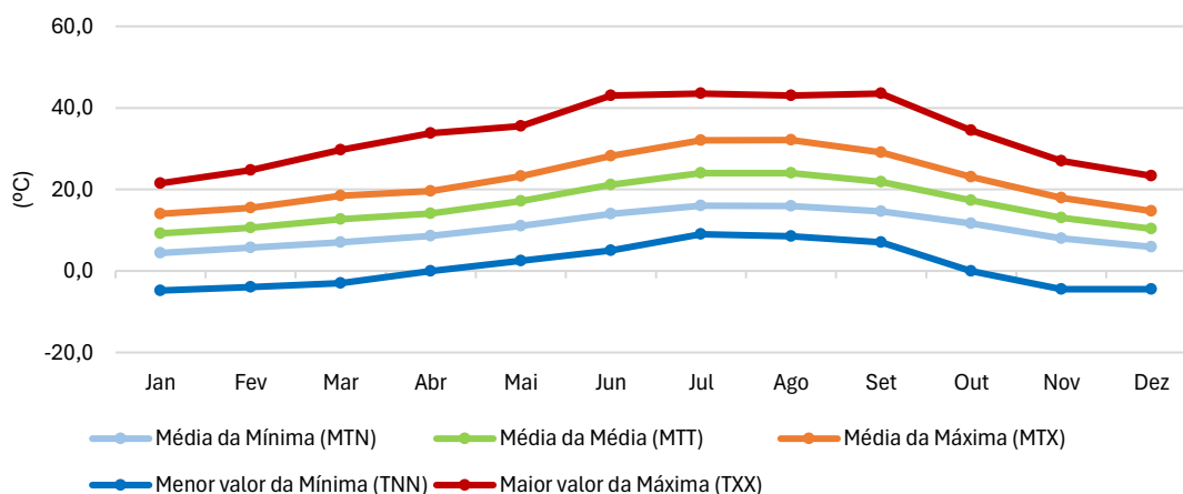
Figura 29. Temperatura do ar segundo as normais climatológicas para o período 1971-2000 | Estação Meteorológica de Benavila
