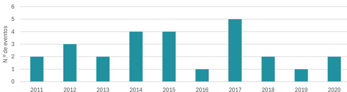
Figura 54. Número de eventos de ondas de calor, por ano (2010-2020) | Estação Meteorológica de Portalegre Fonte: IPMA
