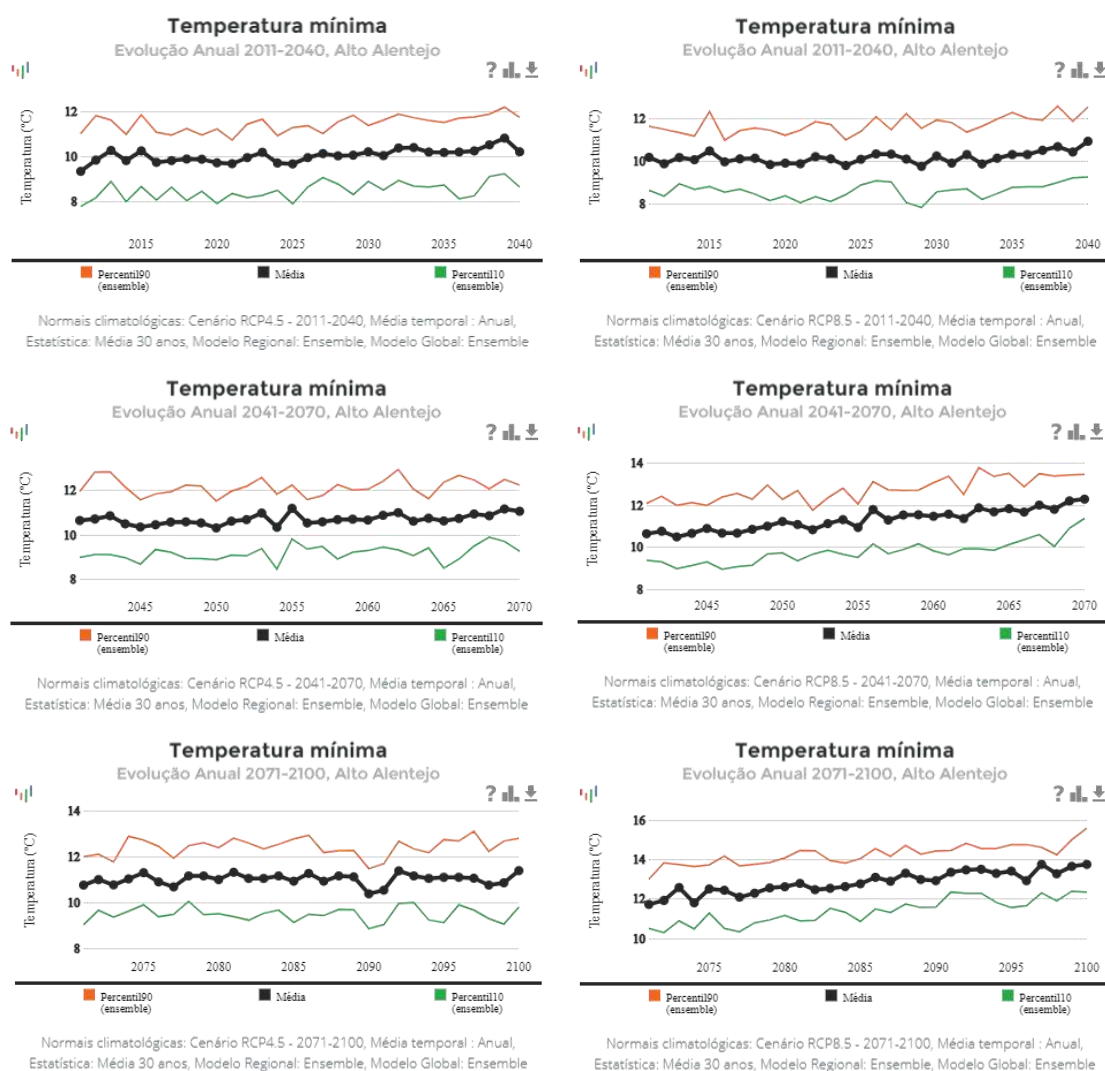
Figura 34. Projeção das anomalias climáticas (médias) da temperatura mínima - para os períodos 2011-2040, 2041-2070 e 2071-2100 - cenário RCP4.5 (à esquerda) e cenário RCP8.5 (à direita)
